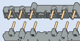
Соединительный комплект, UW для использования с устройством взаимной блокировки ► см. стр. 82
