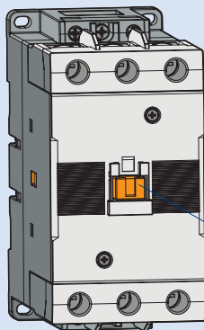
Блок вспомогательных контактов, UA1 Установка сбоку, 1 ЗК+1 РК ► см. стр. 77
