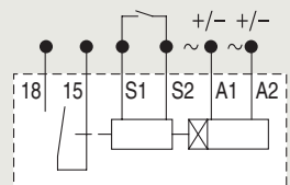
Электрическая схема
