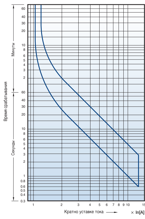
Холодный пуск
