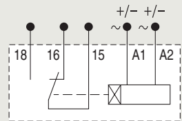
Электрическая схема
